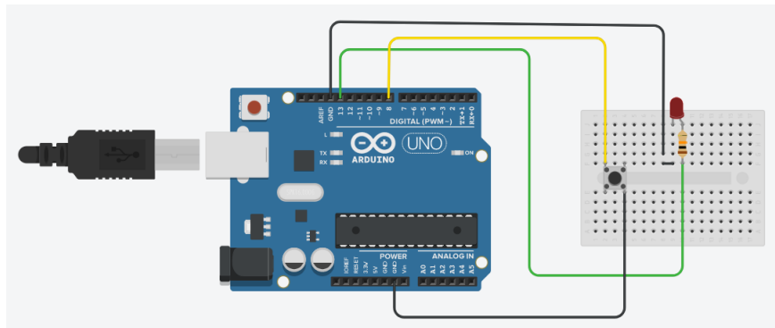
Fig. 2.6 Schema electrică pentru citirea stării unui buton.
